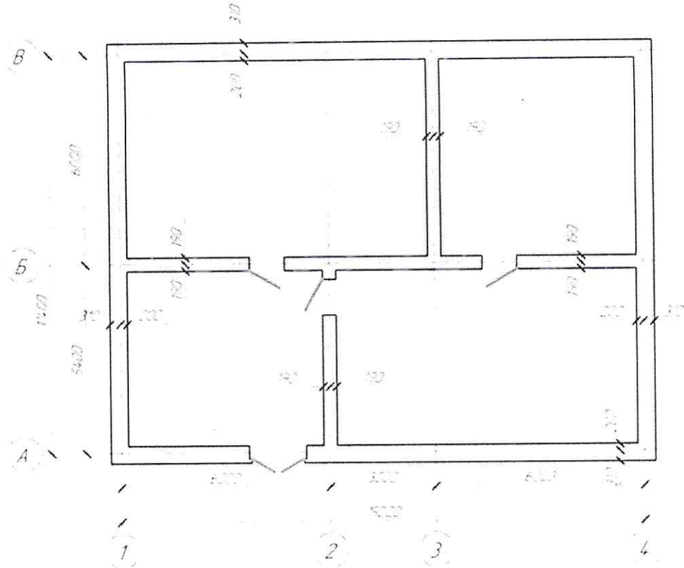
Рисунок 1. Кладочный чертеж к заданию 1 Модуля 2
